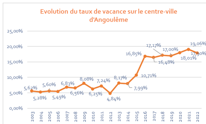
Graphique – L'évolution du taux de vacance sur le centre-ville d'Angoulême (Sources : CODATA, Traitement Bérénice)
