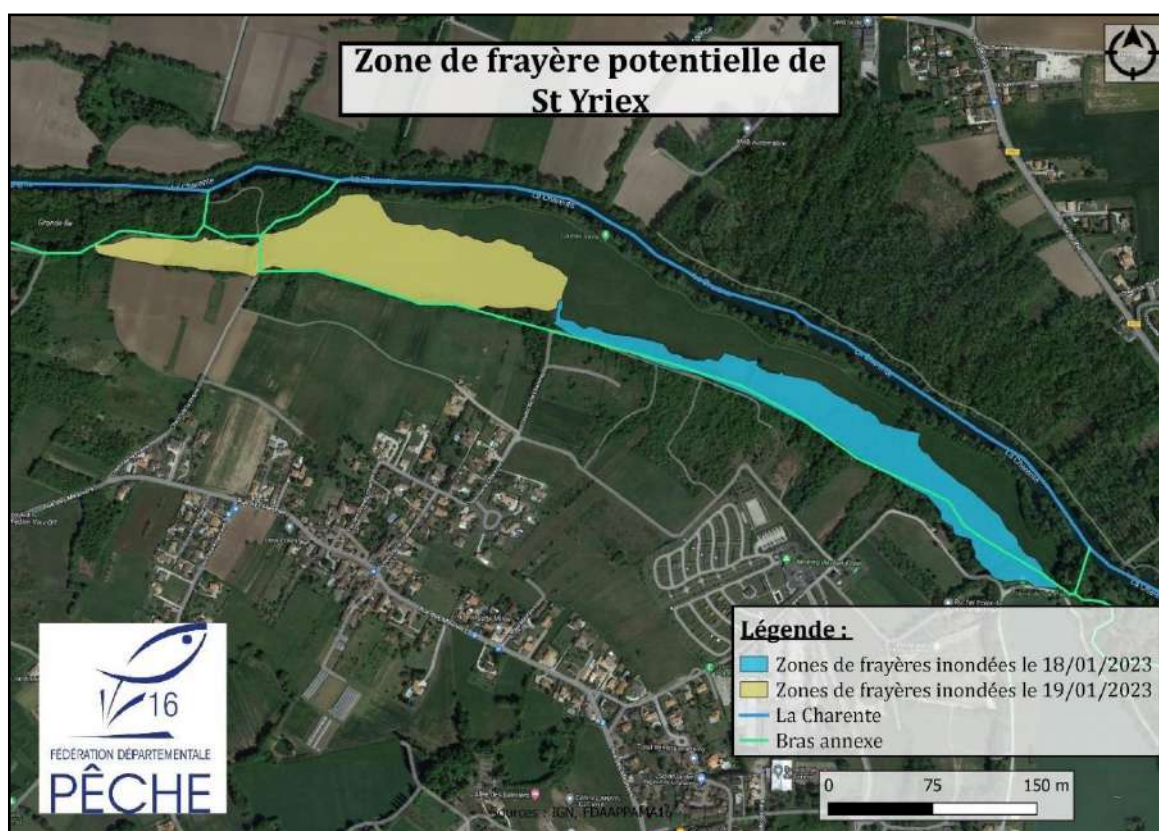
Figure 58 : Zone de frayère potentielle de St-Yrieix-sur-Charente
