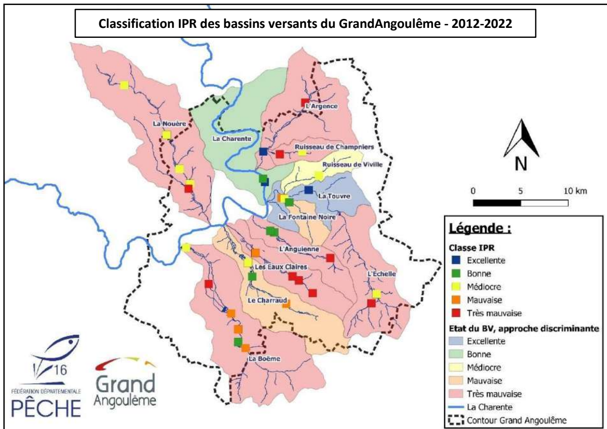
Carte 19 : Classification IPR des bassins versants du GrandAngoulême (données 2012-2022)
