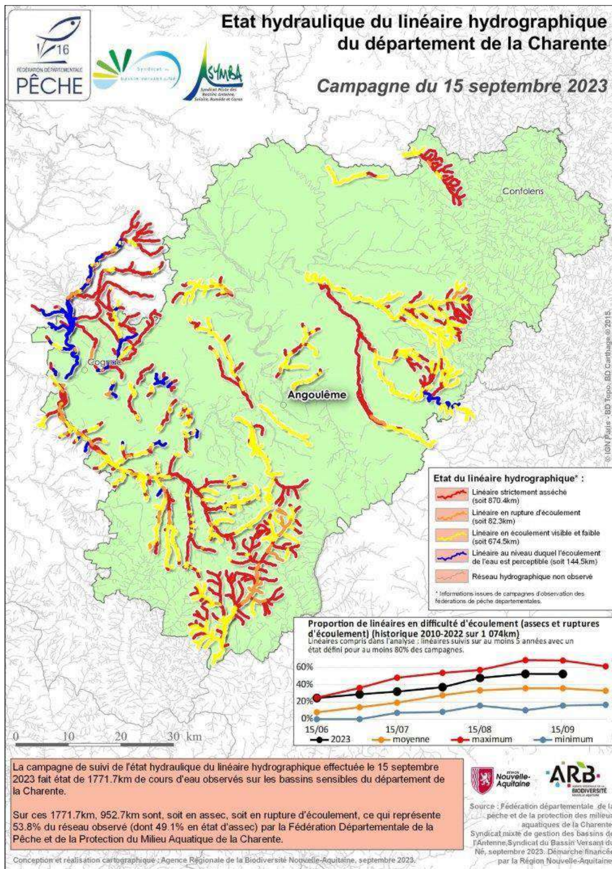
Carte 3 : Suivi des écoulements sur le département de la Charente, campagne du 15 septembre 2023
