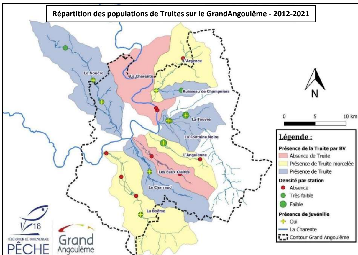
Carte 21 : Répartition des populations de Truites fario sur le GrandAngoulême (données 2012-2021)
